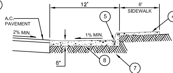
SEC. A-A
